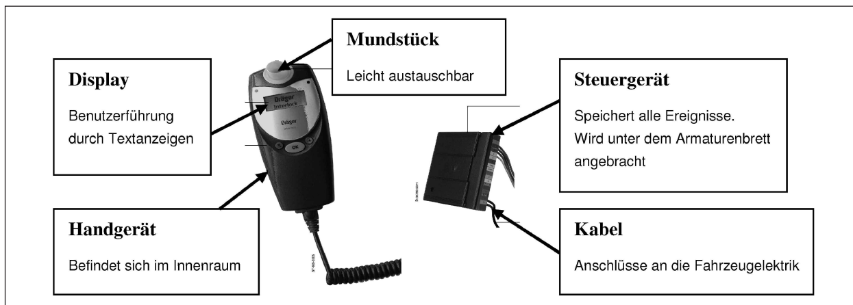
Bild 1: Beispiel eines Alkohol-Interlocks (mit freundlicher Genehmigung der Firma Dräger)
